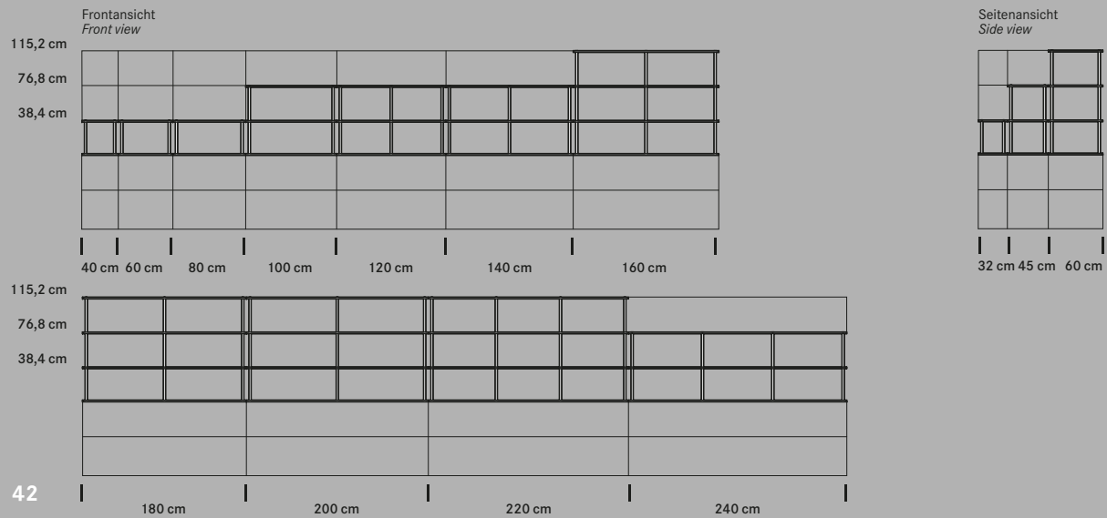
WINEA MAXX offene Aufsatzregale WINEA MAXX open top shelves
