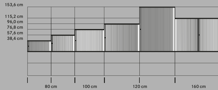
Querrolladenaufsätze, 1-4 Ordnerhöhen Upper tambour door parts, 1-4 file heights
