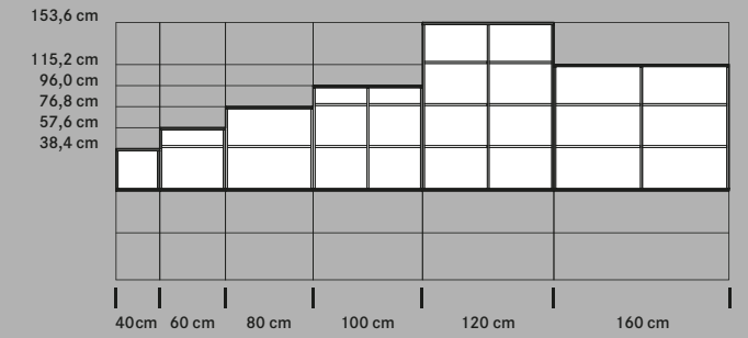
Schiebetürsaufsätze, 1-4 Ordnerhöhen Upper sliding door cabinets, 1-4 file heights
