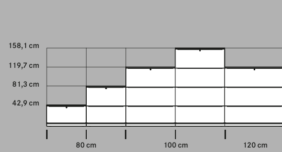
Hängehefterschränke, 1-3 Ordnerhöhen Hanging file cabinets, 1-3 file heights
