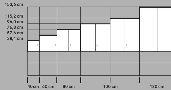
Querrolladenaufsätze, 1-4 Ordnerhöhen Upper tambour door parts, 1-4 file heights
