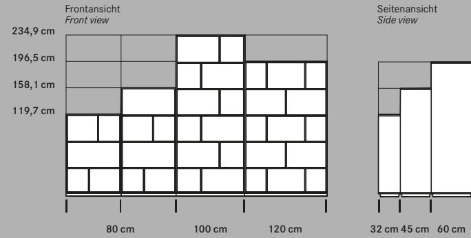
Flügelürsaufsätze, 1-4 Ordnerhöhen Upper double door cabinet parts, 1-4 file heights
