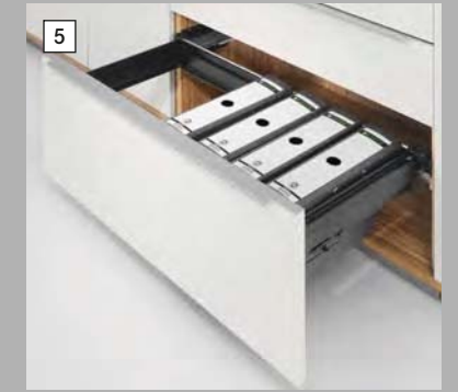
5 Hängeregisterauszug mit stabiler, zahnradgeführter Parallelführung.
