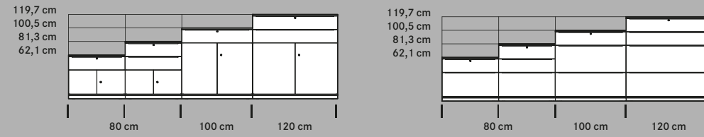
WINEA MAXX Regale mit versetzter Mittelseite WINEA MAXX bookcases with asymmetric separation panel
